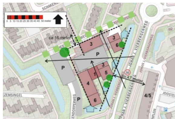
Situatie tekening locatie Schuylenburcht
